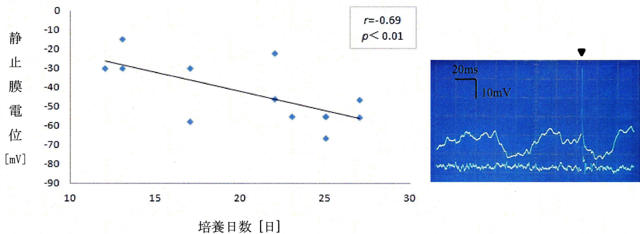
図2 (左) 分化誘導した iPS 細胞の培養日数による静止膜電位の変化 (右) 活動電位 (自発発火: \blacktriangledown ) の記録例 (上: 膜電位変化、下: 膜電流変化)
