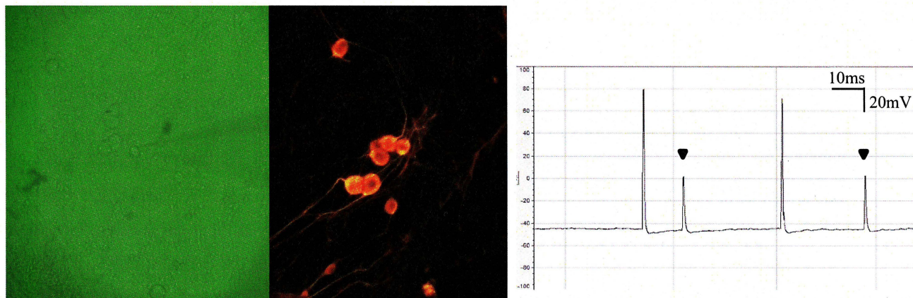
図1 (左) 微小電極を用いたホールセルクランプの例 (中) ホールセルクランプした DRG 細胞の \beta III-tubulin による免疫染色結果 (右) 活動電位 (自発発火: \blacktriangledown ) の記録例 (無印は外部印加による膜電位変化)
