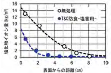
遮塩性試験結果の例
