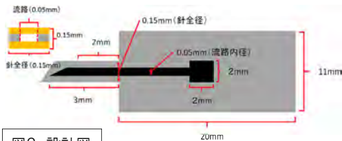
図2 設計図
